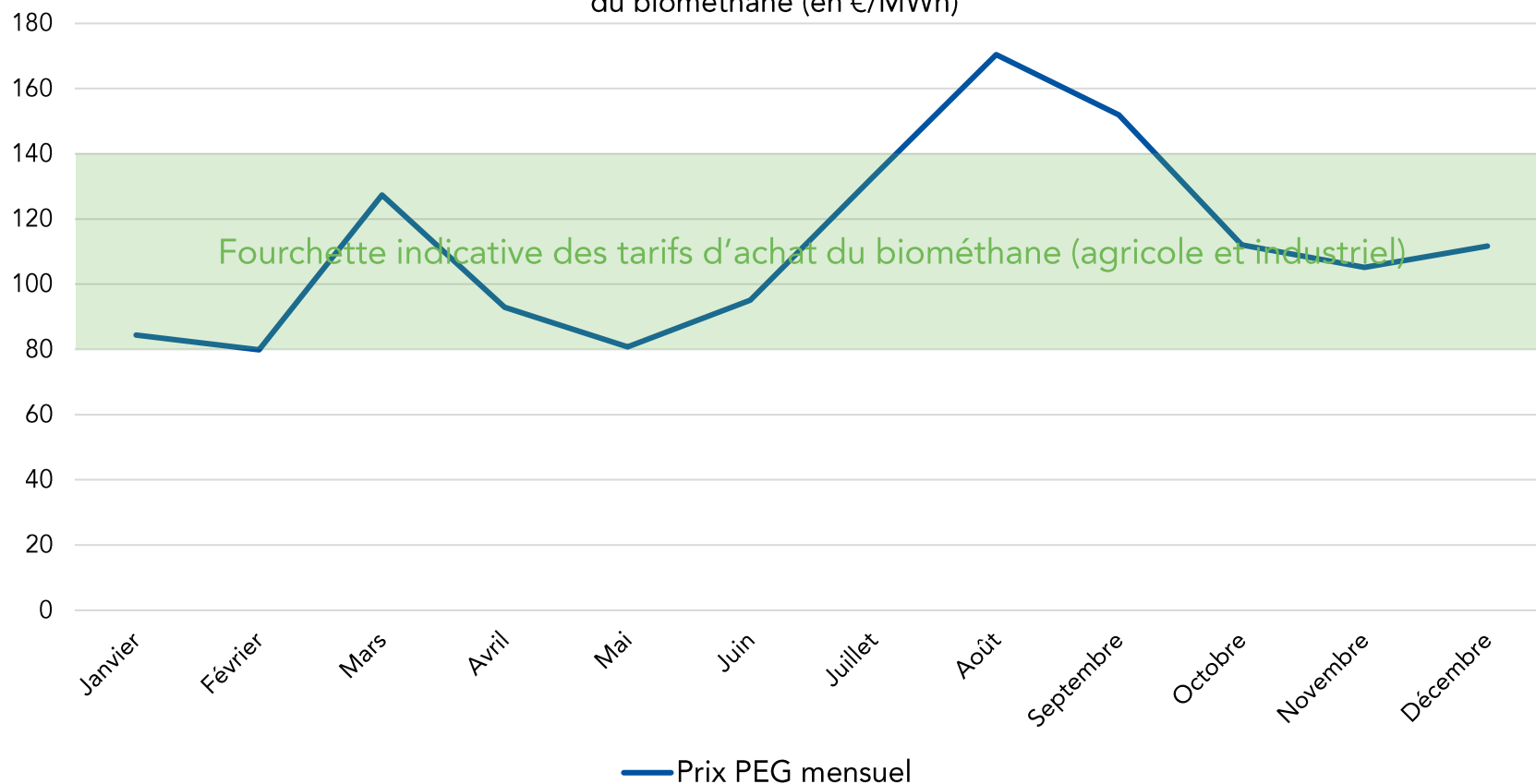
Comparaison des prix de marché du gaz naturel en 2022 (PEG) et des tarifs d'achat réglementés du biométhane (en €/MWh)
