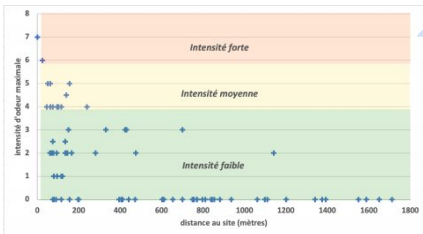
Intensités d'odeurs en fonction de la distance aux unités, cumul sur les 5 unités
